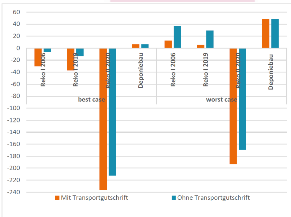
Abbildung 2: Treibhausgaspotenzial der Verwertungsoptionen mit und ohne Gutschrift für den vermiedenen Transport der Primärmaterialien aus dem Ausland in die Niederlande; Quelle Fraunhofer IWKS 17
